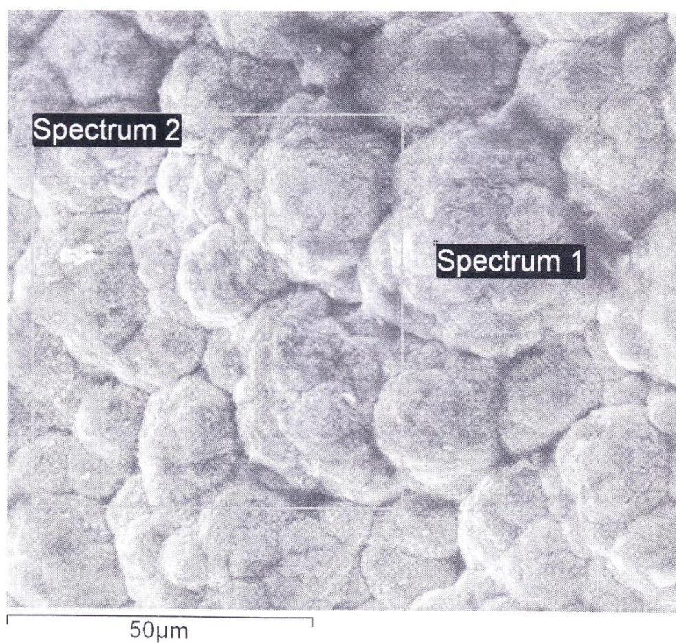
Рис. 7. Микроструктура покрытия фильтрующего элемента с иллюстрацией мест локального химического анализа (увеличение \times 1200 )
