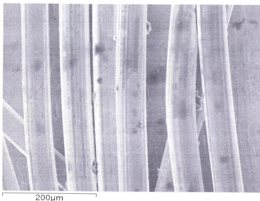
Рис. 1. Микрофотография проволоки (увеличение ×200)
