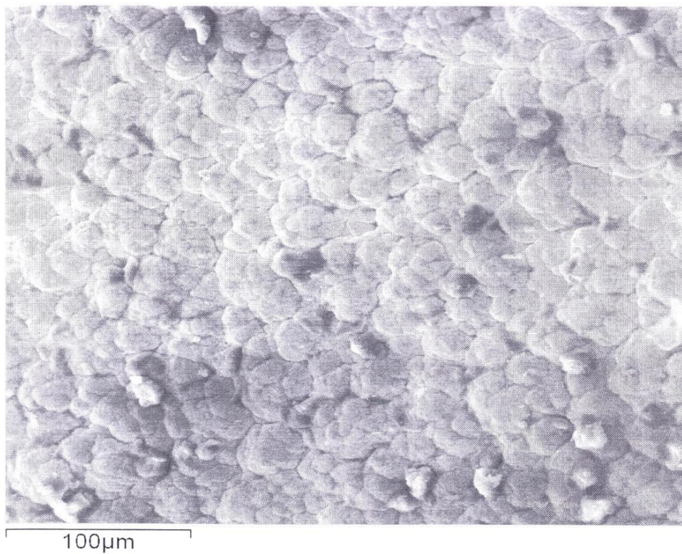
Рис. 6. Микроструктура поверхностного слоя (покрытия фильтрующего элемента)
