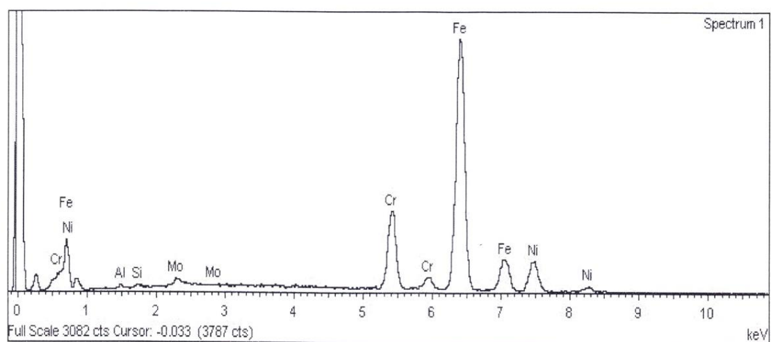
Рис. 3. Спектрограмма содержания химических элементов в проволоке (первая локальная точка поверхности)
