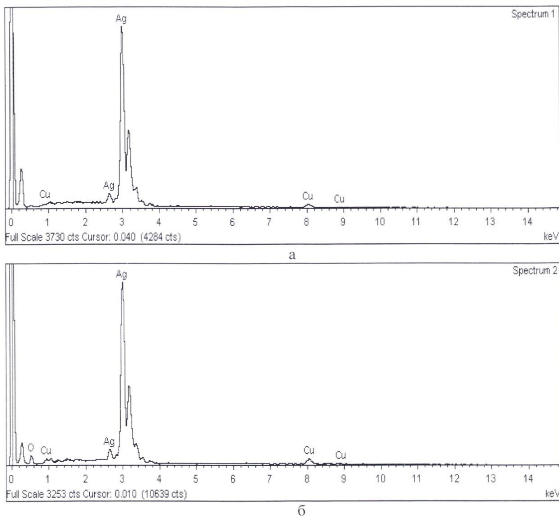
Рис. 8. Спектрограммы содержания химических элементов (а) в локальной точке; (б) на локальной площади поверхности корпуса фильтрующего элемента
