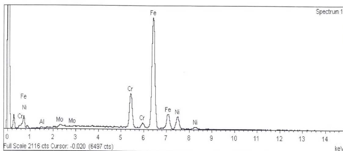
Рис. 5. Спектрограмма содержания химических элементов во второй локальной точке проволоки
